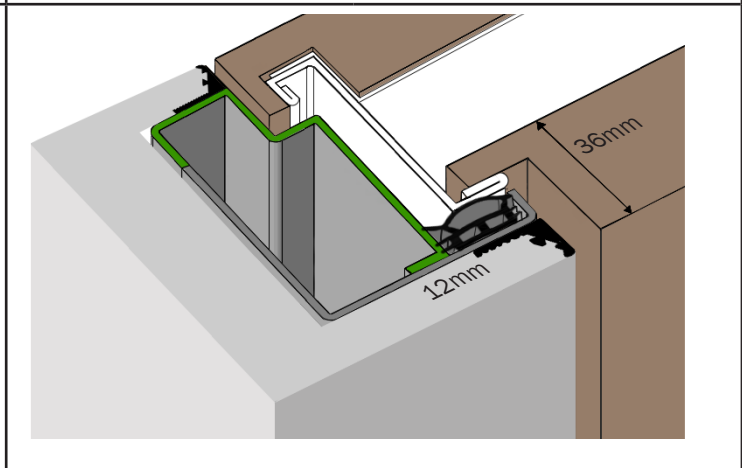
COMPLANARITA' ESTERNA
