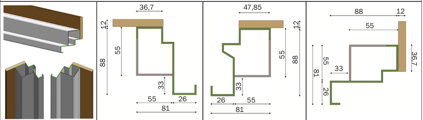
TELAIO SSAV (CON MOSTRINE COPRIFILO)
