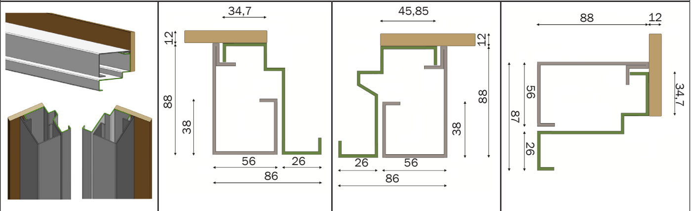
TELAIO A SCORRERE (CON MOSTRINE COPRIFILO)
