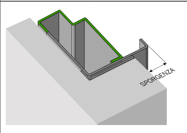
SOLUZIONE CON ALETTA GUIDA INTONACO
