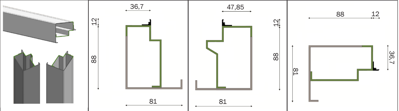
TELAIO TAGLIO TERMICO (CON MOSTRINE COPRIFILO)
