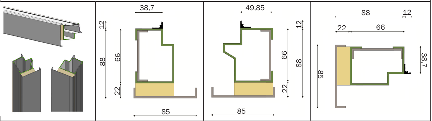
TELAIO TAGLIO TERMICO FILOMURO (CON PROFILI GUIDA INTONACO)
