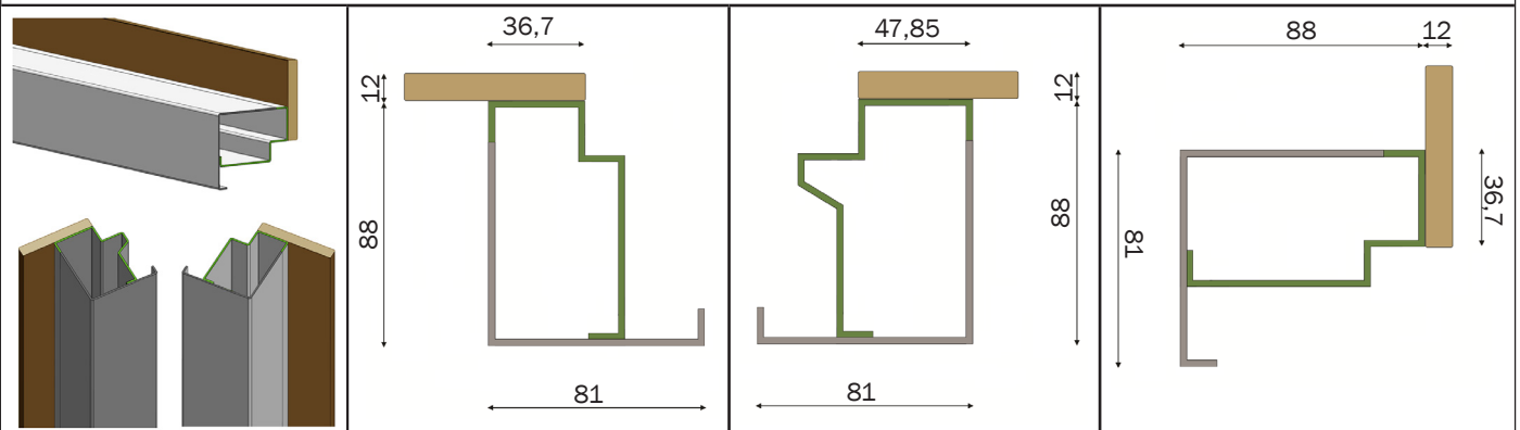
TELAIO A SCORRERE FILOMURO (CON PROFILI GUIDA INTONACO)
